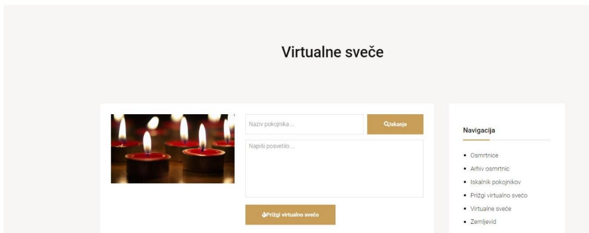
Slika 1: Virtualna svečka
